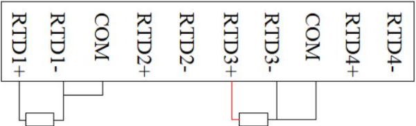
2线制接法 RTD-和COM短接
